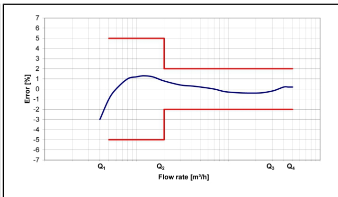
Tipikus hibagörbe
